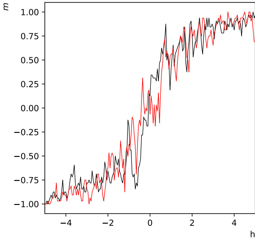
Hystérésis de l'aimantation réseau de taille L=8 - h=5 à T=5
