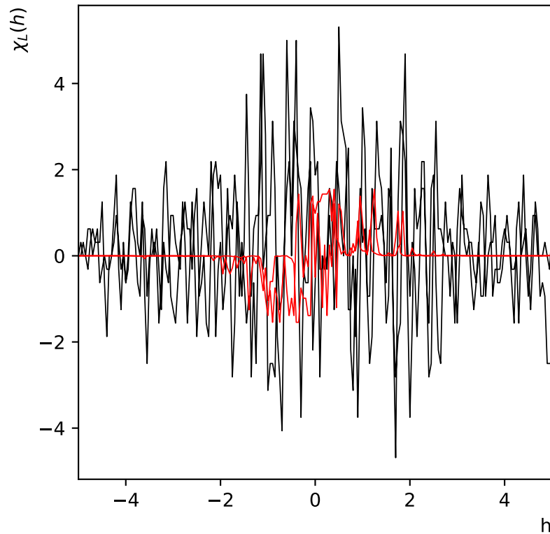
\chi_L(h) réseau de taille L=8 à T=5
